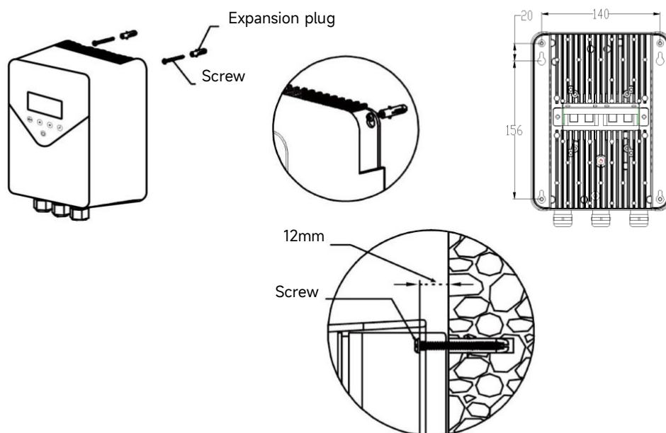
Abb.3 Montagediagramm für Wandaufhängungen
