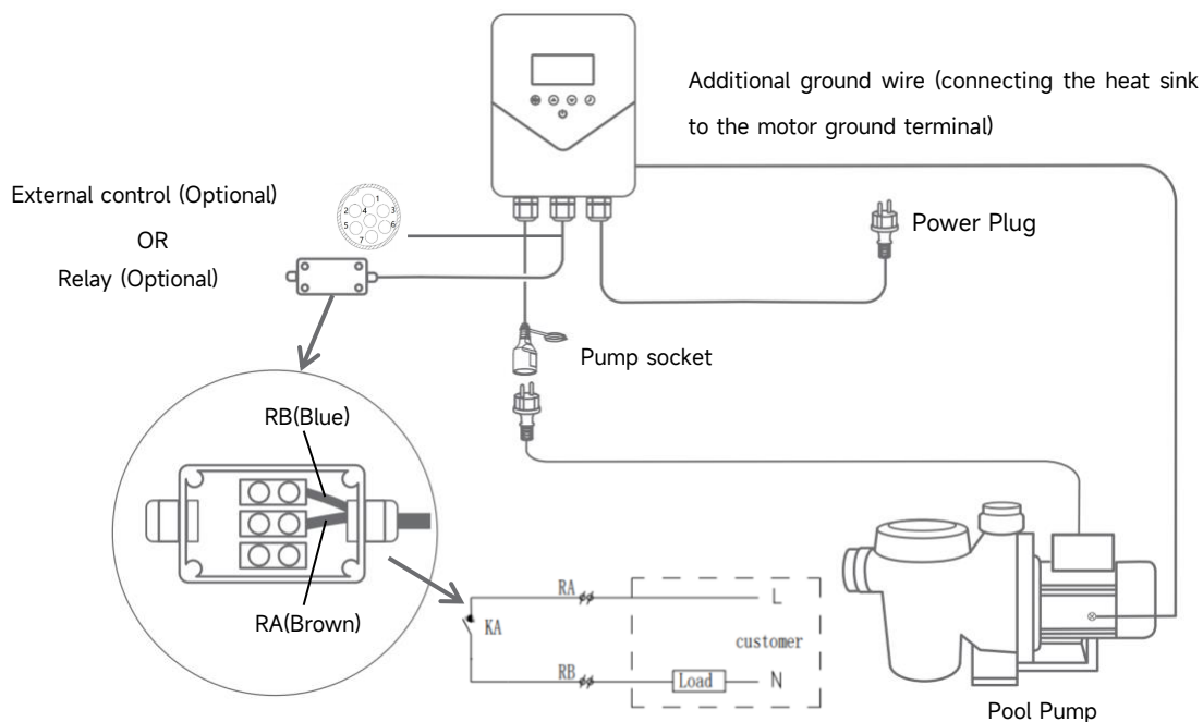
Abb.4 Kabelanschlussplan
