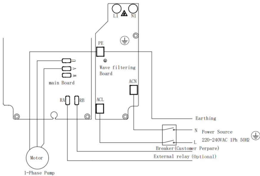
Feige.6 1-PH Pumpenanschlussplan
