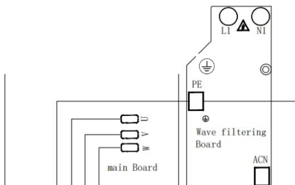
Feige.6 1-PH Pumpenanschlussplan
