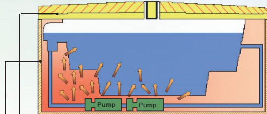
Wärmedämmsystem
